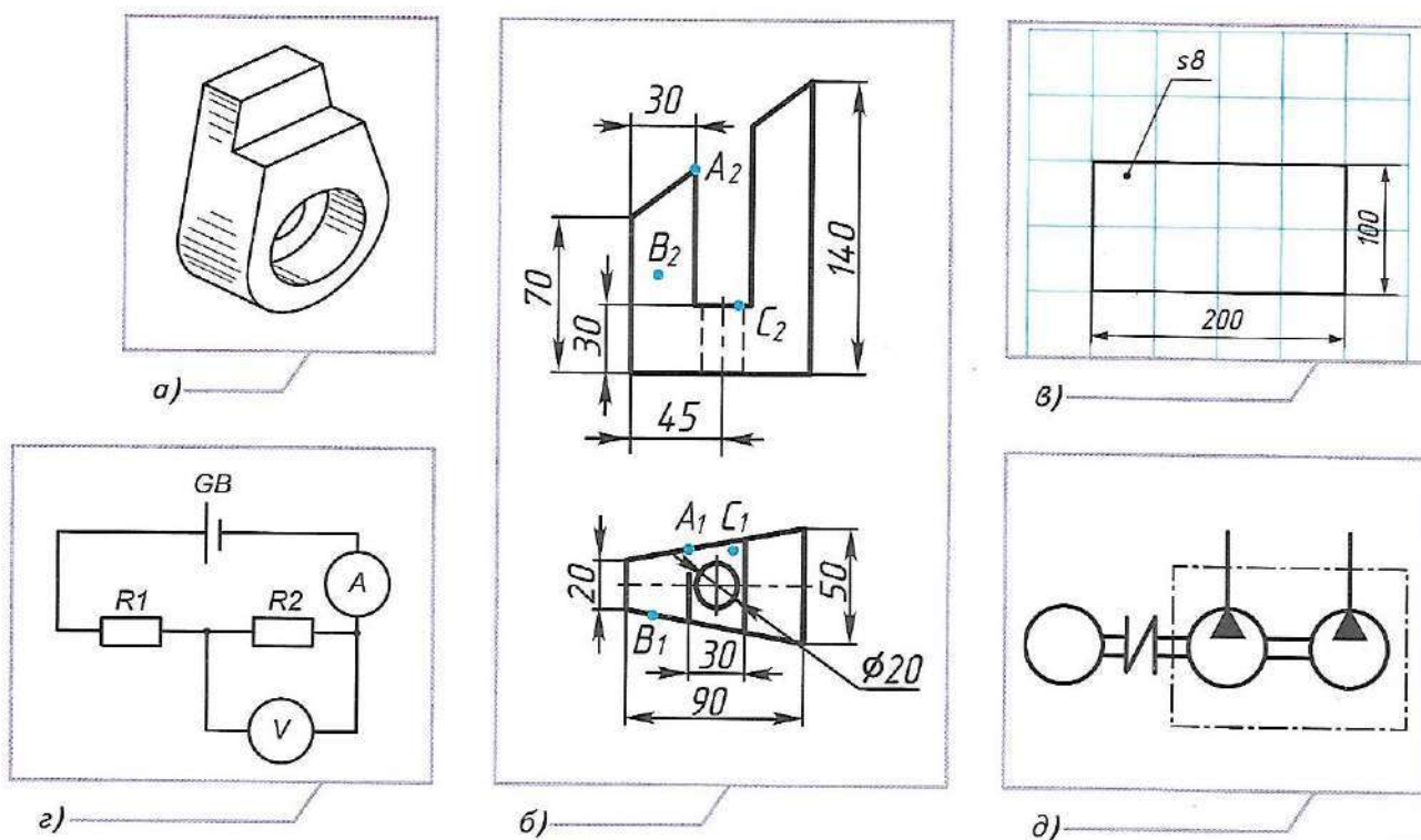
Рис. 3.4. Конструкторская документация: а — технический рисунок; б — чертёж; в — эскиз; г — электрическая схема; д — пневматическая схема
