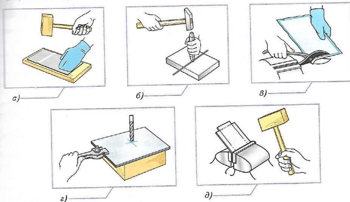
Рис. 5.3. Технологии обработки металлов ручными инструментами: а — правка; б — рубка; в — разрезание и отрезание; г — сверление; д — гибка
