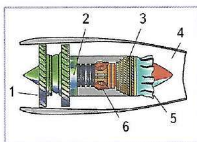
Рис. 9.9. Реактивный двигатель: 1 — вентилятор; 2 — компрессор; 3 — турбина; 4 — сопло; 5 — смеситель; 6 — камера сгорания
