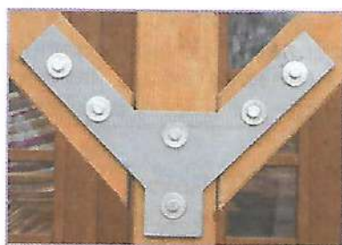
Рис. 6.4. Крепление деталей из древесины на болтах
