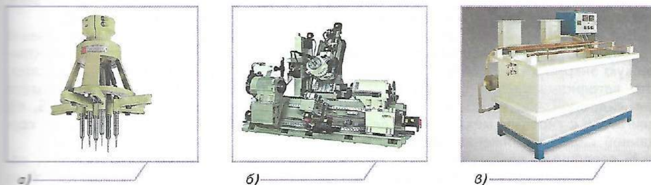
Рис. 4.4. Рабочий орган многошпиндельного сверлильного станка (а); токарно-фрезерный обрабатывающий центр (б); гальваническая установка для нанесения электрическим током покрытий на металлы (в)
