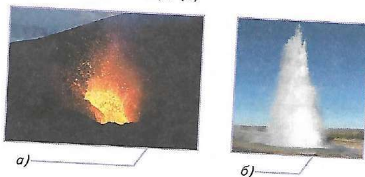
Рис. 9.3. Извержение вулкана (а) и гейзера (б)
