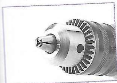
Рис. 5.10. Патрон для крепления свёрл (а); образцы свёрл (б); наиболее распространённые виды свёрл (в): 1 — спиральное; 2 — витое; 3 — перьевое
