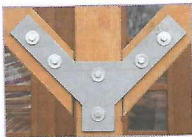
Рис. 6.4. Крепление деталей из древесины на болтах
