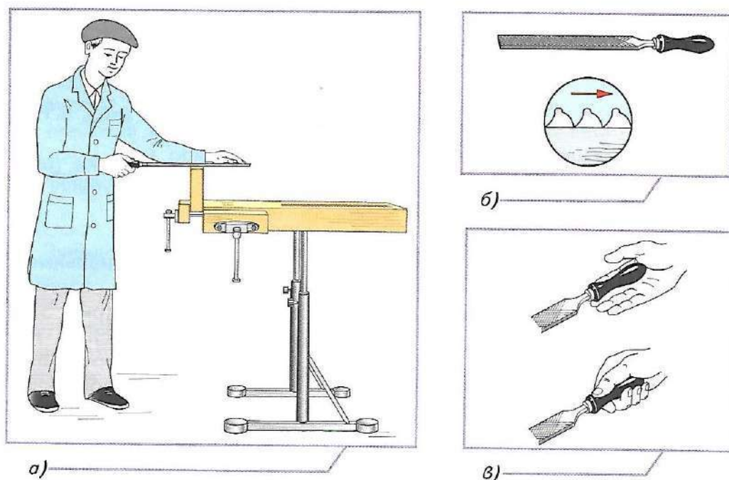
Рис. 5.18. Опиливание: а — рабочая поза при опиливании сходна с рабочей позой при зачистке деревянных поверхностей; б — конструкция напильника; в — хватка напильника
