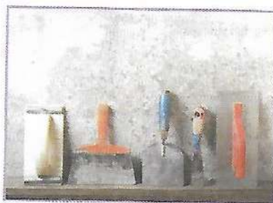
Рис. 7.6. Наружное оштукатуривание: а — выравнивание штукатурки тёркой; б — виды кельм и тёрок; в — разбрызгиватель штукатурки
