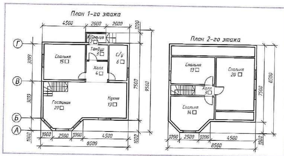
Рис. 3.5. Пример строительного чертежа
