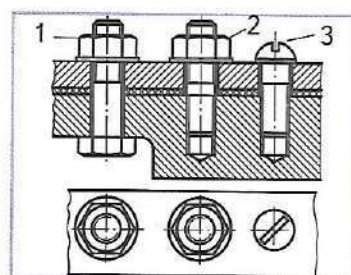
Рис. 6.5. Основные виды резьбовых соединений
