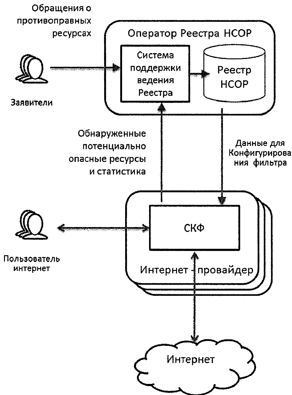
Рисунок 6. Принцип контроля доступа через Реестр НСОР
